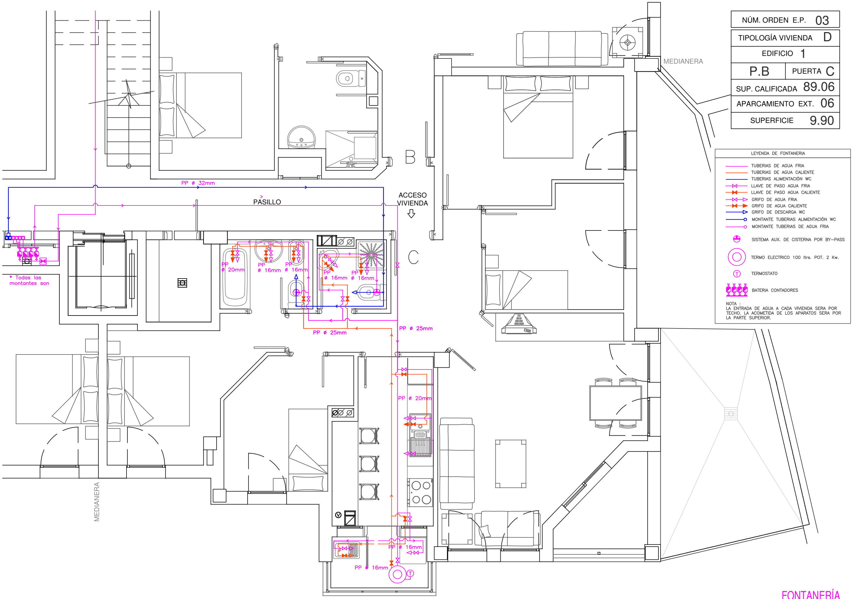
62 VIVIENDAS DE PROTECCIÓN PÚBLICA EN PEGUERA CALVIÀ - PLANTA BAJA - E:1/50
