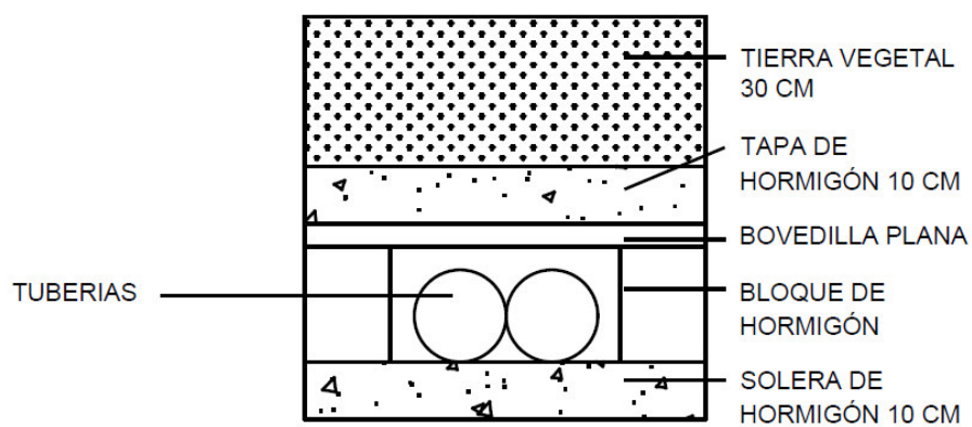
DETALLE DE ZANJA 70 X 70 CM
