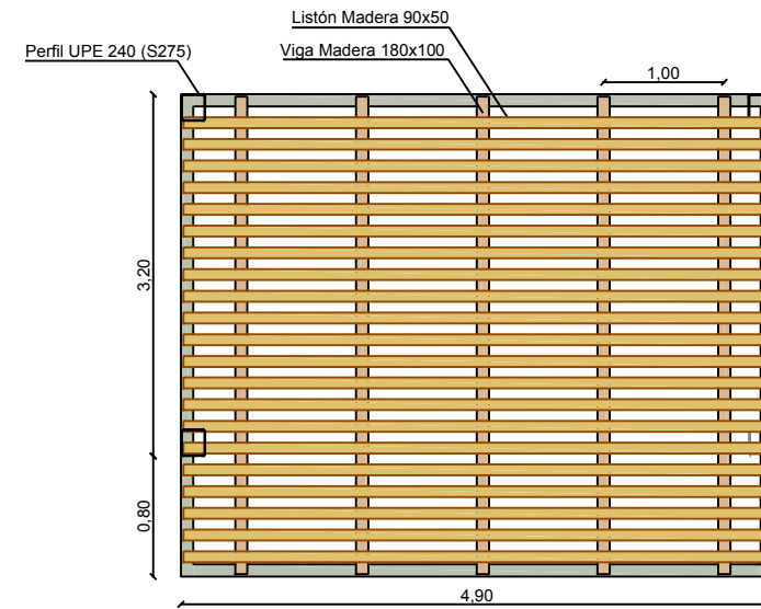
PLANTA TIPO E:1/50
