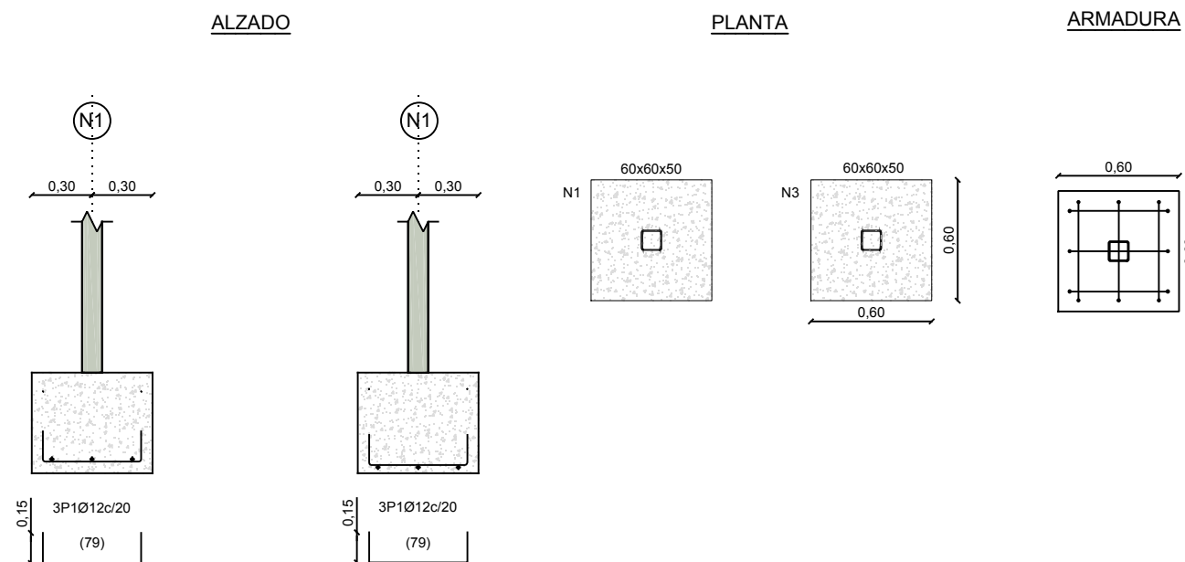
DETALLE ARMADO ZAPATA E:1/25
